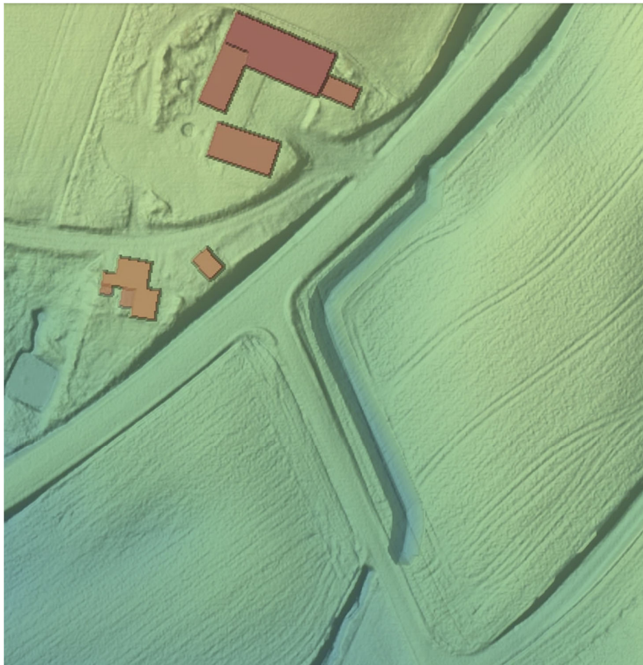
Etablering af det nye vandløbstracé langs Skyumvej og Østerstrandsvej. Udklip fra Scalgo.
